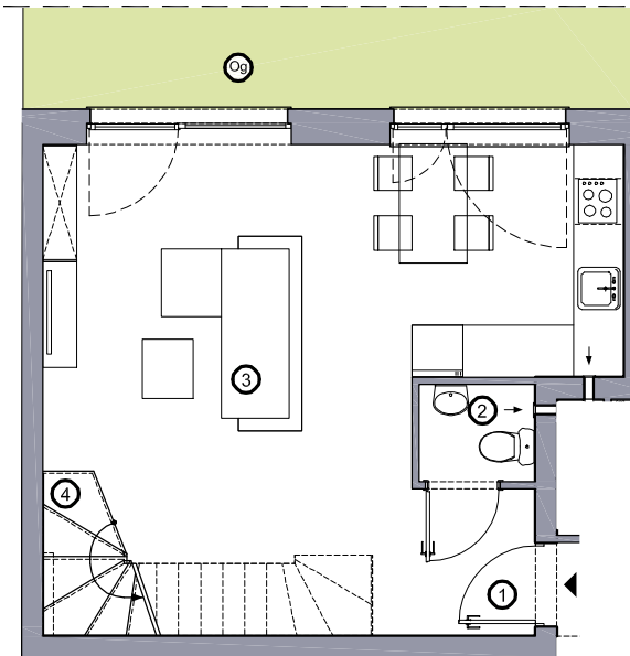
Rzut parteru
