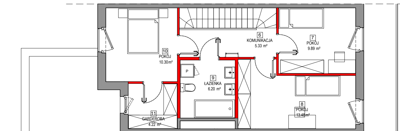
PIĘTRO
