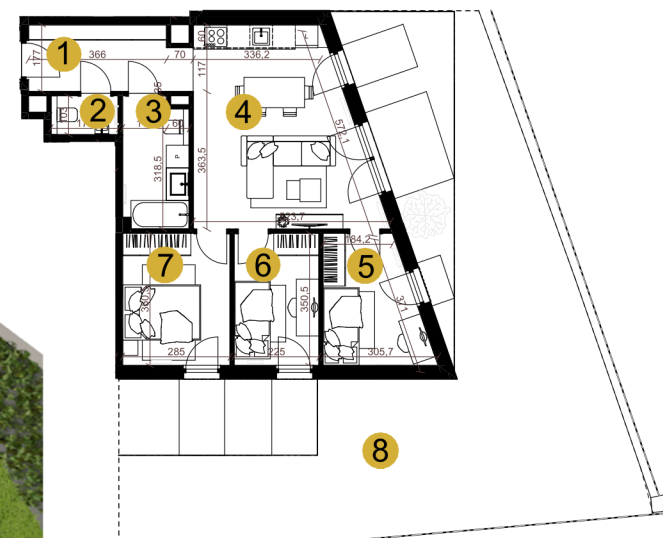
Rzut kondygnacji
