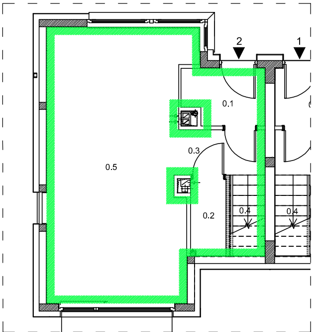
RZUT PARTERU BUDYNKU NR 11G LOKAL MIESZKALNY NR 2
