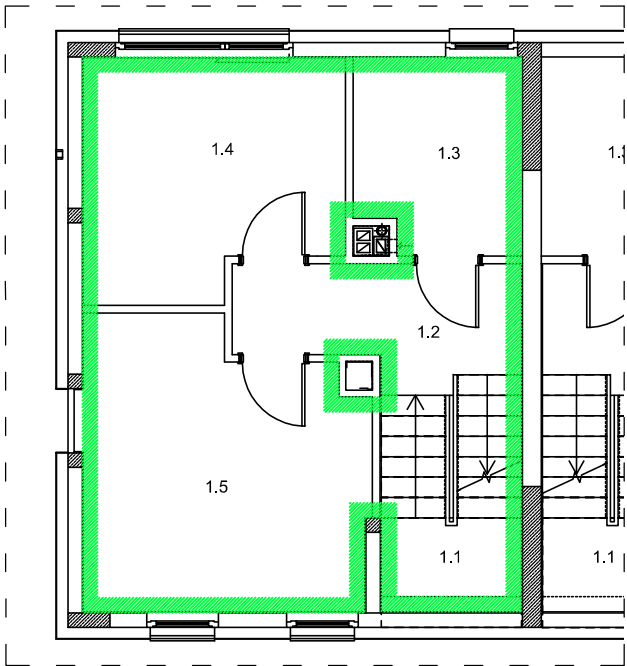
RZUT PIĘTRA I-GO BUDYNKU NR 11G LOKAL MIESZKALNY NR 2
