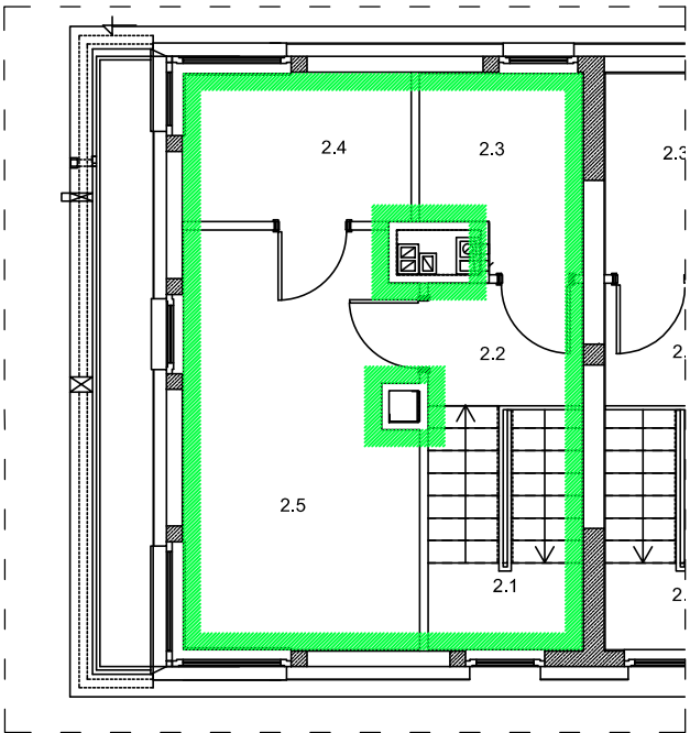
RZUT PIĘTRA II-GO BUDYNKU NR 11G LOKAL MIESZKALNY NR 2
