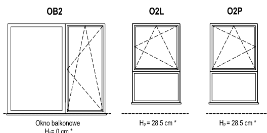
SCHEMAT OKIEN W WIDOKU OD ZEWNĄTRZ
