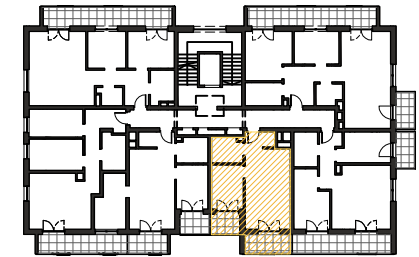
Schemat kondygnacji +4
