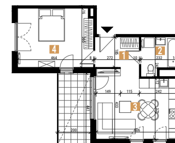
Rzut mieszkania
