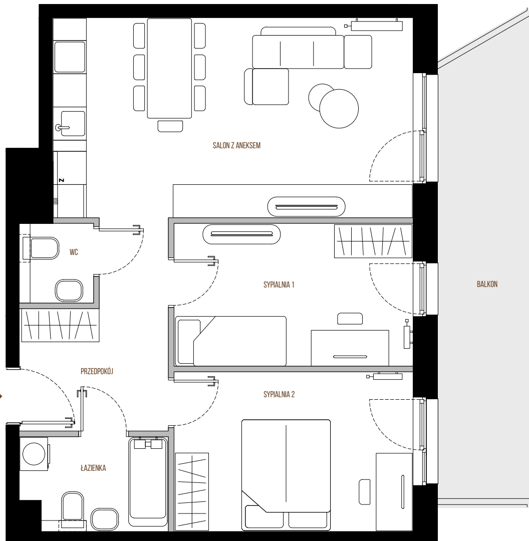
RZUT LOKALU
