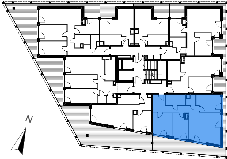
PIĘTRO 1 MIESZKANIE A.06
