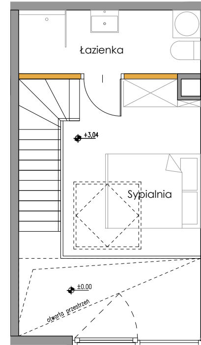
RZUT PIĘTRA
