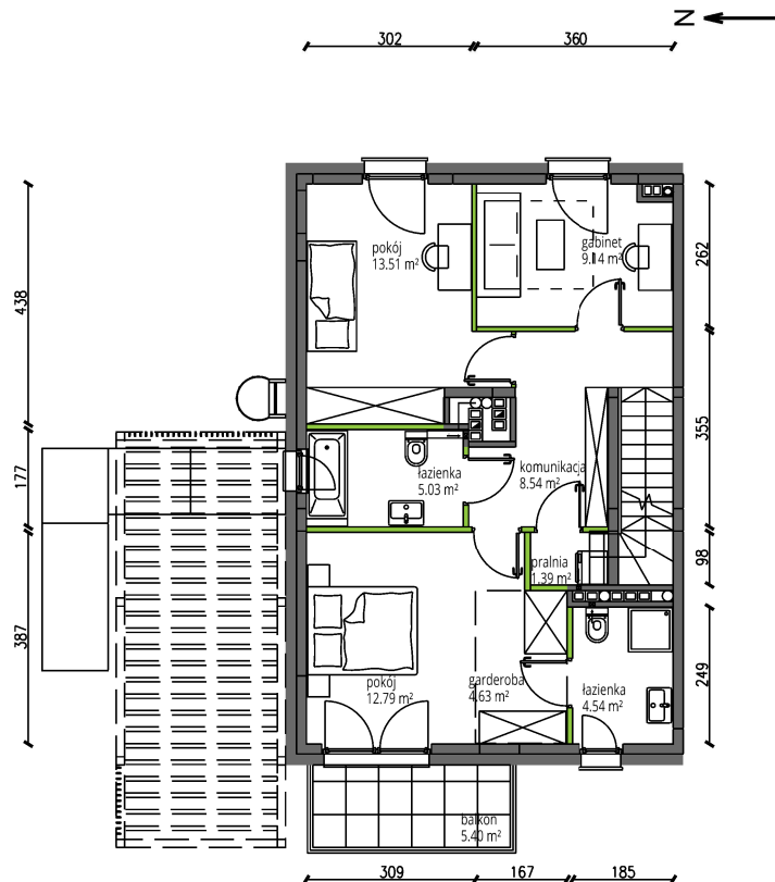
II PIĘTRO
