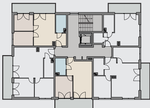
RZUT KONDYGNACJI
