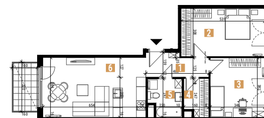
Rzut mieszkania
