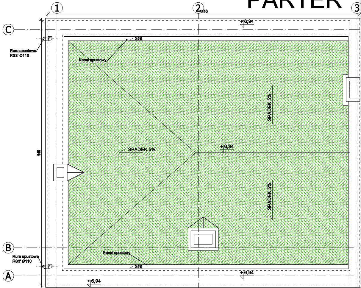
DACH
