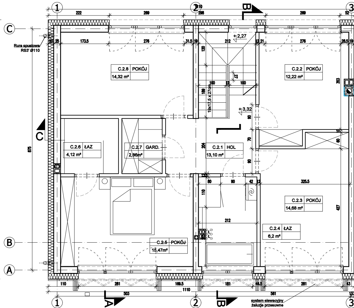
PIĘTRO
