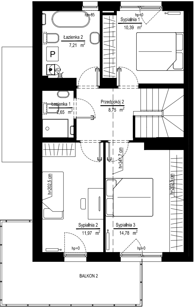
RZUT KONDYGNACJI
