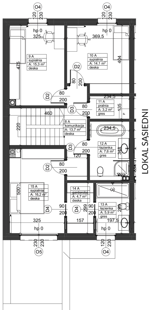
rzut piętra
