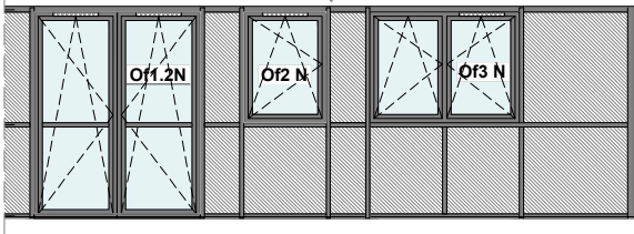
schemat okien w widoku od zewnątrz
