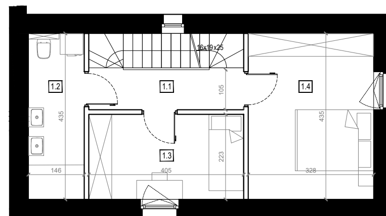
PIĘTRO I
