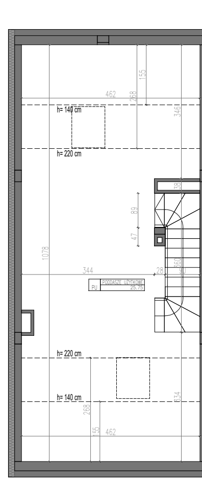
PODDASZE UŻYTKOWE
