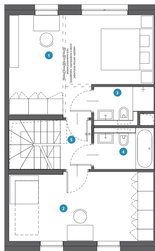
RZUT 1 PIĘTRA
