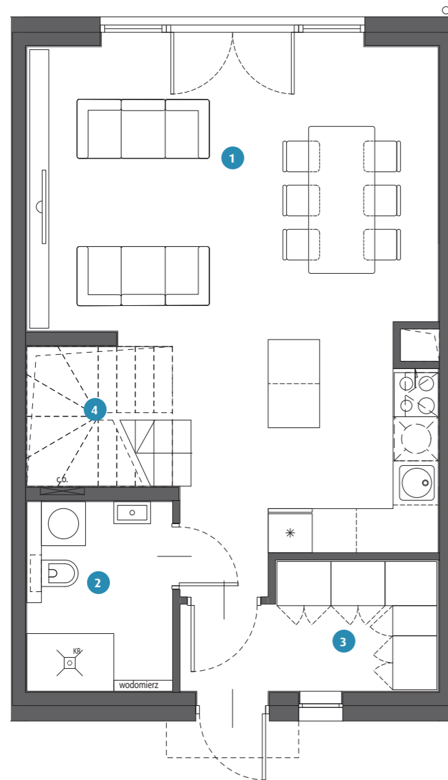
RZUT PARTERU
