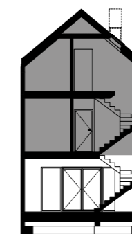
Przekrój
