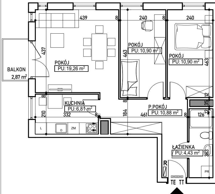
RZUT KONDYGNACJI 2 PIĘTRA BUD. A Z ZAZNACZENIEM LOKALU MIESZKALNEGO
