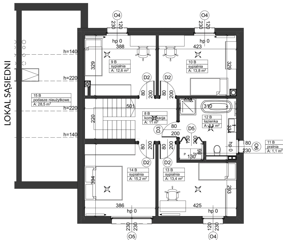
rzut piętra
