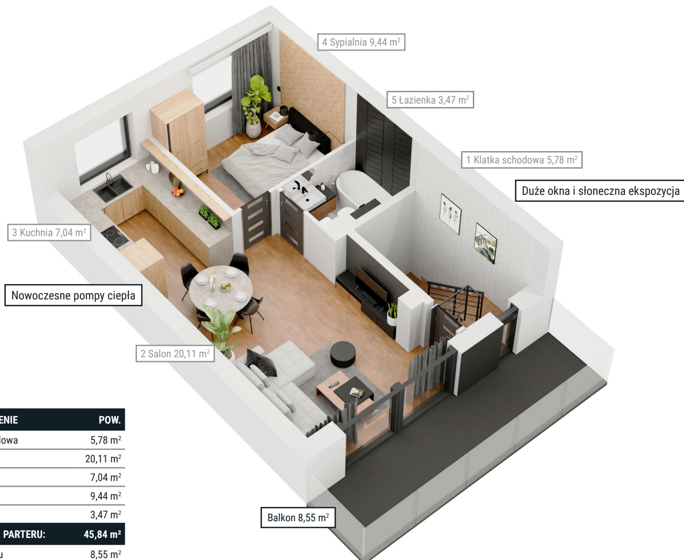
Rzut parteru
