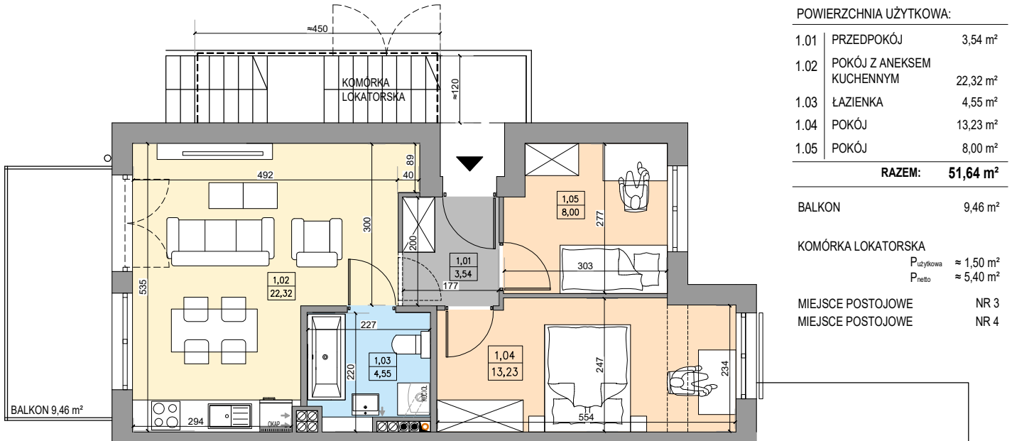
RZUT LOKALU NA PIĘTRZE
