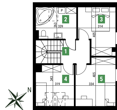
Rzut poddasze
