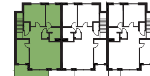
RZUT 2 PIĘTRA
