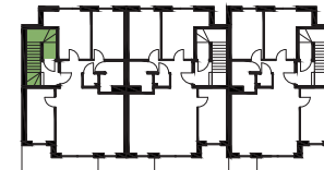
RZUT 1 PIĘTRA
