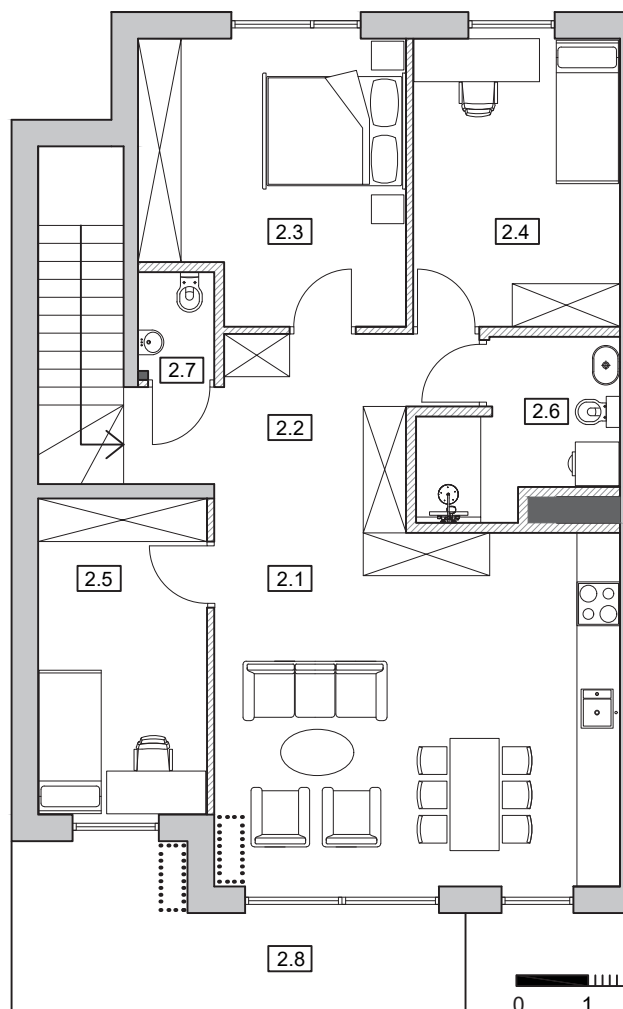
RZUT 2 PIĘTRA
