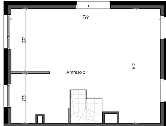
Rzut antresoli
