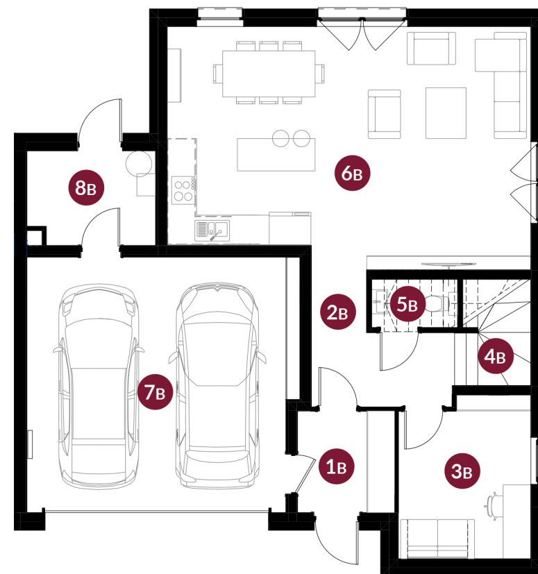
rzut parteru
