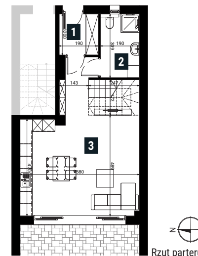
Rzut parteru
