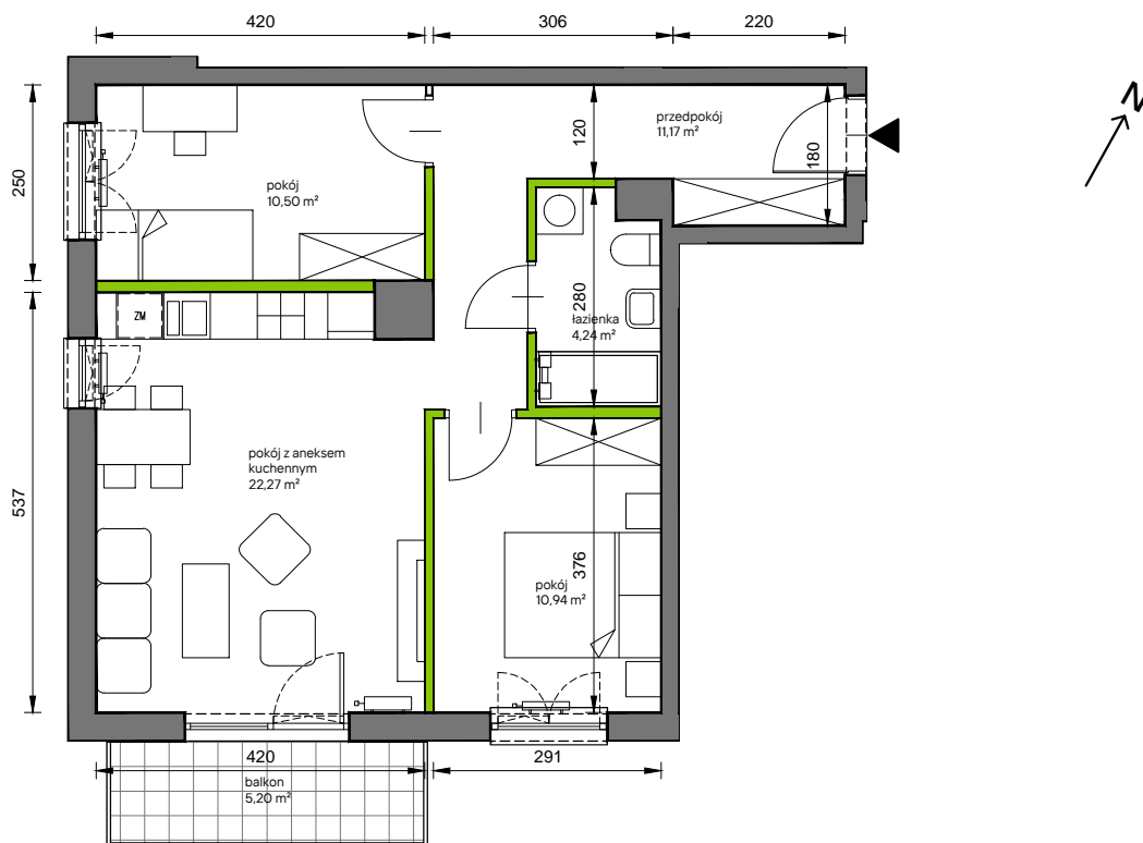
Rzut kondygnacji Piętro 2
