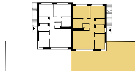
RZUT KONDYGNACJI
