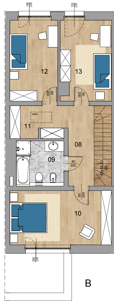
RZUT 1 PIETRA
