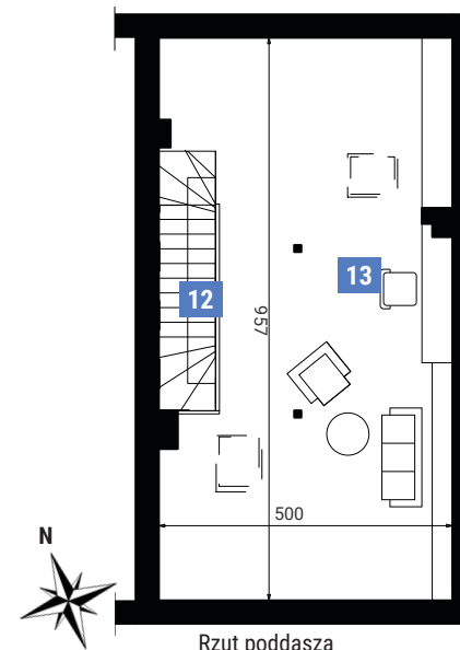
Rzut poddasza
