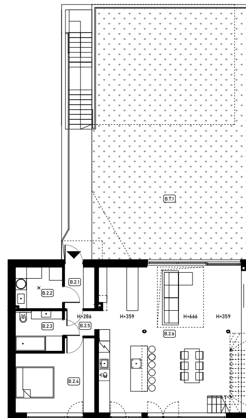
POZIOM 1
