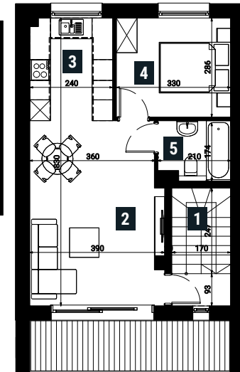
Rzut apartamentu
