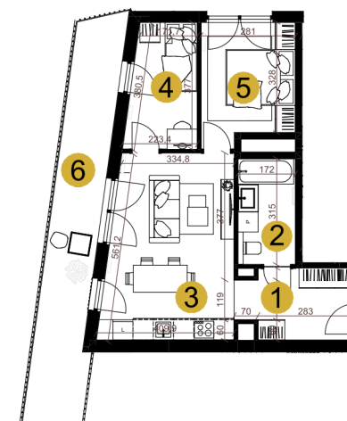
Rzut kondygnacji
