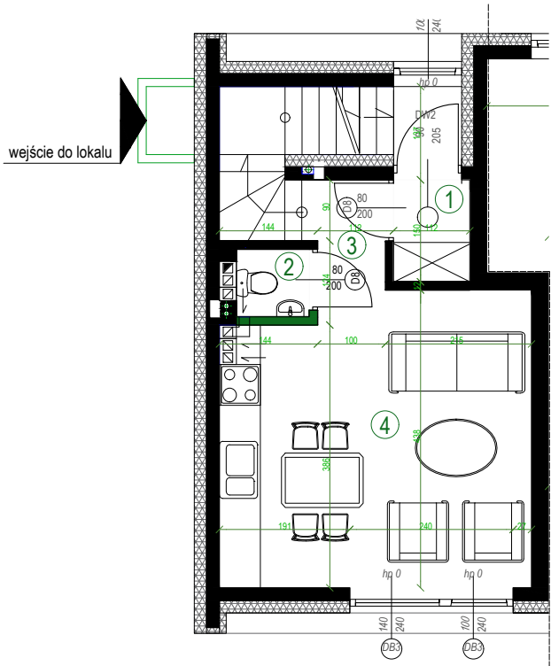
I PIĘTRO
