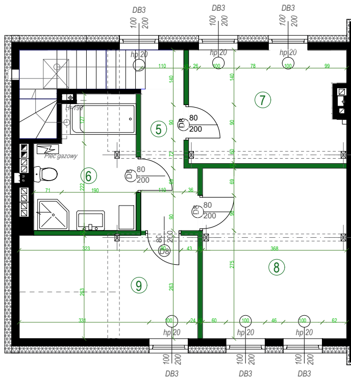
II PIĘTRO
