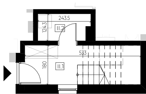
Rzut parteru
