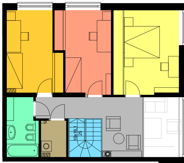
PIĘTRO
