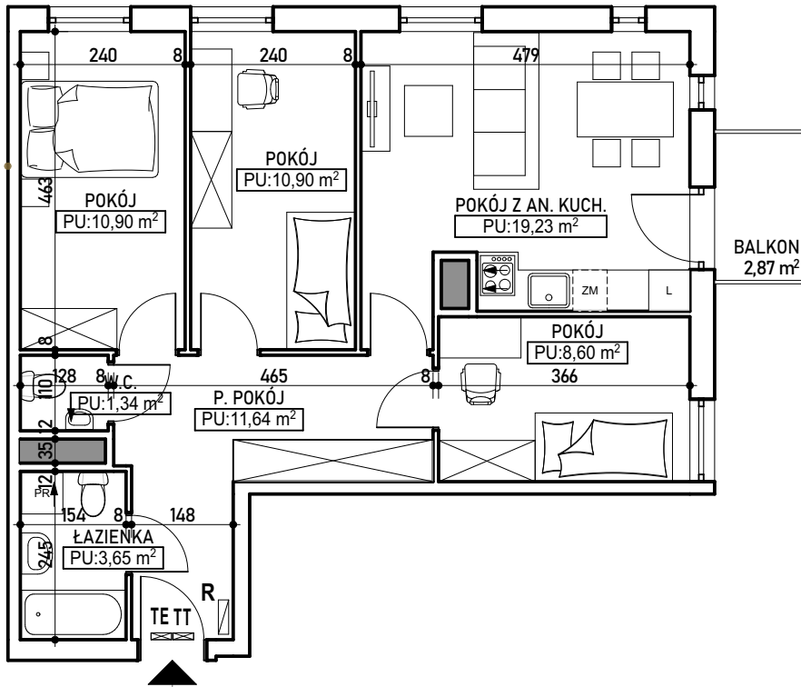
RZUT KONDYGNACJI 3 PIĘTRA BUD. B Z ZAZNACZENIEM LOKALU MIESZKALNEGO
