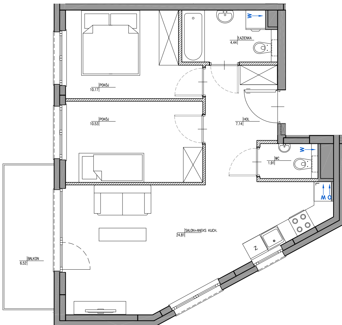
SCHEMAT LOKALU NA RZUCIE
