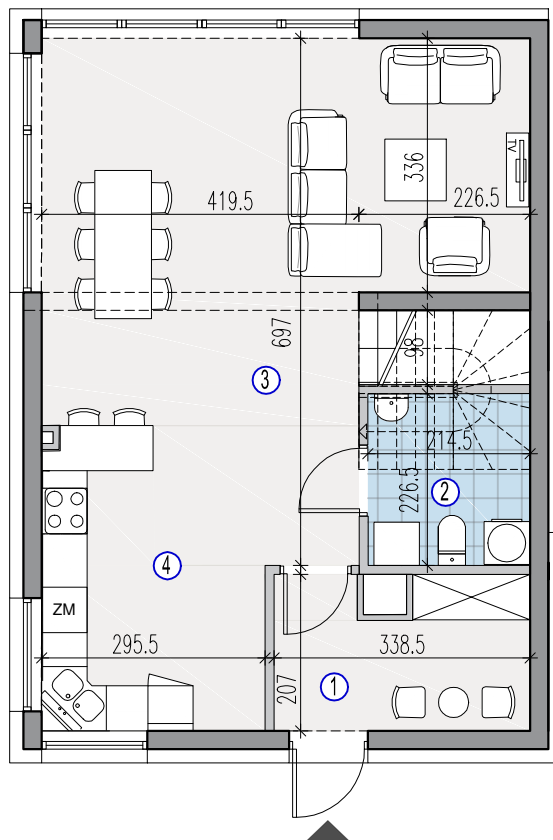
POZIOM +1
