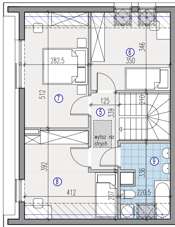
POZIOM +2
