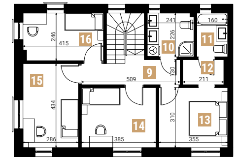
Rzut piętra
