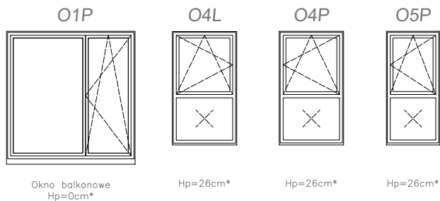
Schemat okien w widoku od wewnątrz:
