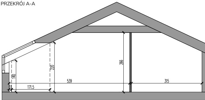
PRZEKRÓJ A-A
