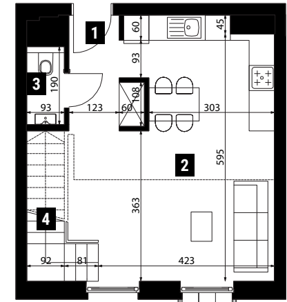
Poziom 0
