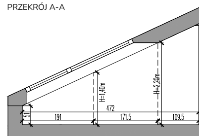
PRZEKRÓJ A-A
