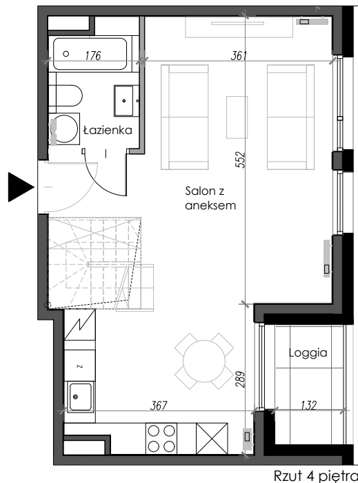
Rzut 4 piętra
