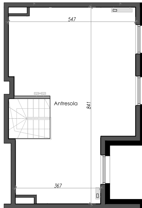
Rzut antresoli
