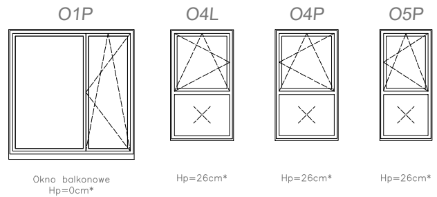
Schemat okien w widoku od wewnątrz:
